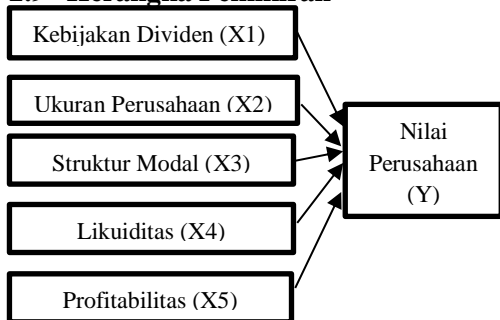
Gambar 1. Kerangka Pemikiran
