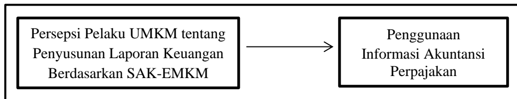
Gambar 1. Kerangka konseptual
